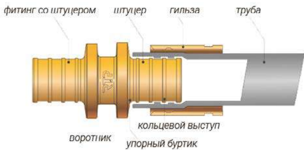
Рис. 3. Элементы аксиальных фитингов ТМ RTP
